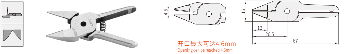
金属尖头平嘴钳 Sharp straight blade
