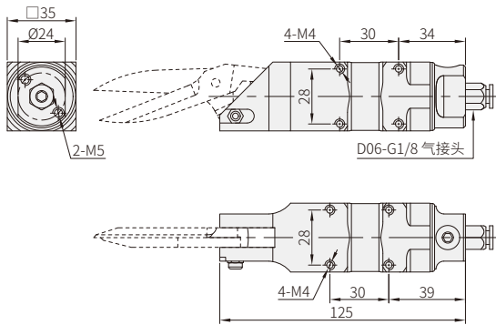
AM-10气剪本体
