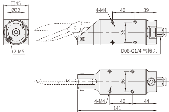
AM-20气剪本体
