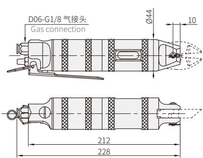
TS-25P气剪本体
