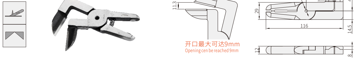
塑胶水口圆头平嘴钳（右拐弯） Straight blade (right)
