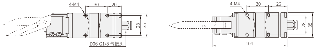
XG-23A气剪本体
