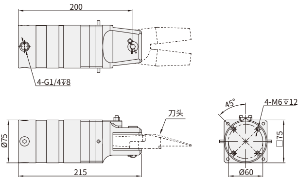
MD-50D气剪本体
