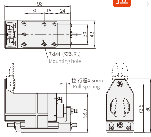
NL-25B气剪本体
