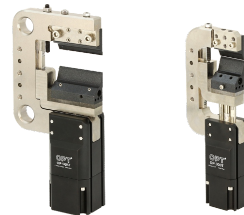
OP-20BTL 左开口 Left shed
