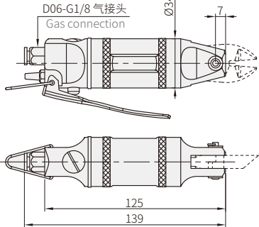
TS-10气剪本体
