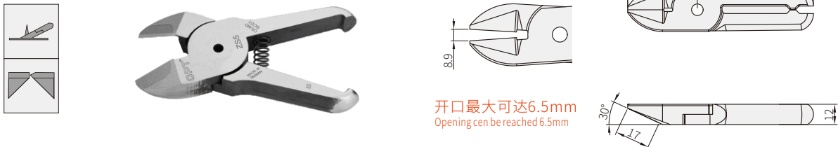
金属圆头斜嘴钳 Bevel blade
