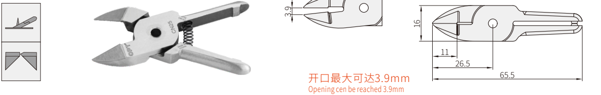
金属尖头斜嘴钳 Sharp bevel blade
