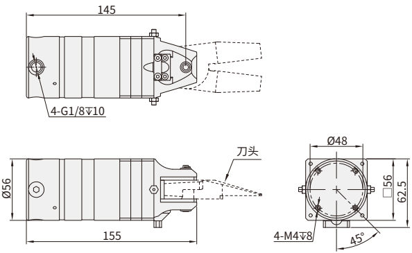
MD-30D气剪本体
