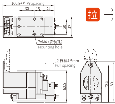
NL-25A气剪本体
