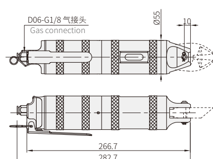
TS-35P气剪本体
