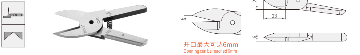
片材剪 Sheet blade
