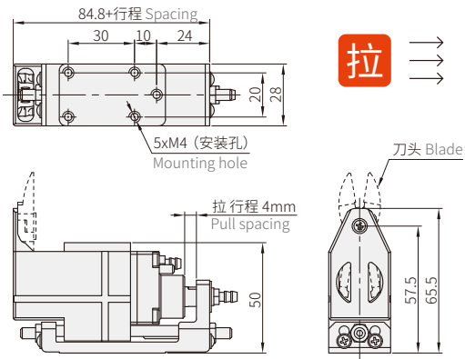
NL-10A气剪本体
