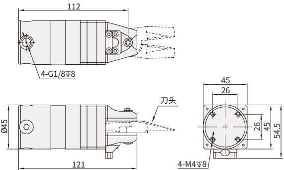
MD-20D气剪本体
