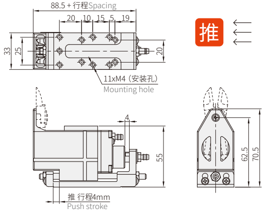
NL-15AR气剪本体
