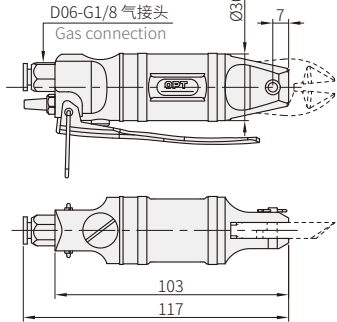
TS-5气剪本体
