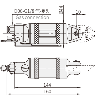
TS-20气剪本体
