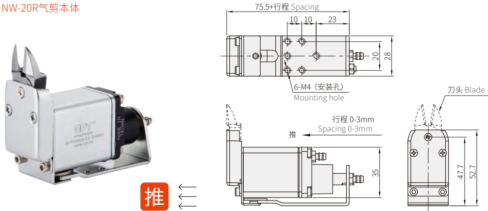
NW-20R气剪本体
