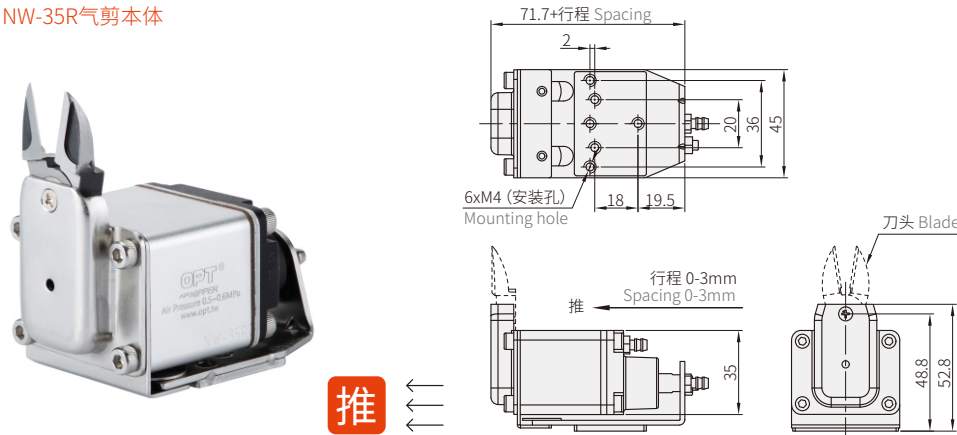
NW-35R气剪本体
