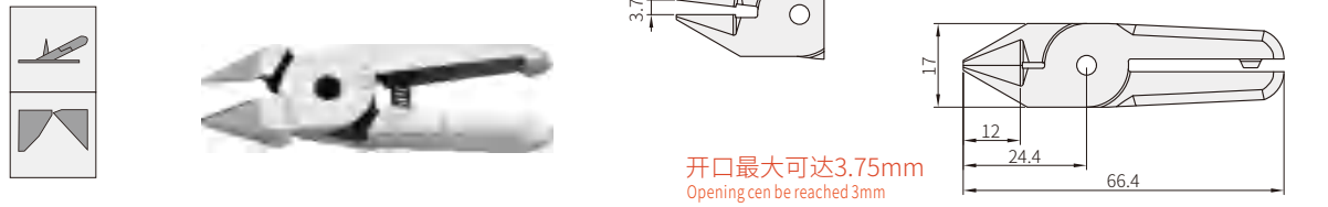
金属尖头斜嘴钳 Bevel blade
