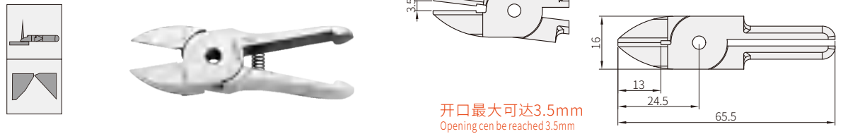
金属圆头平嘴钳 Bevel blade
