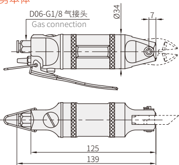
TS-10气剪本体
