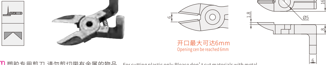
圆头平嘴钳 Round flat edge blade
