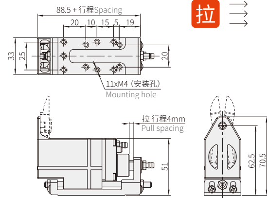
NL-15B气剪本体
