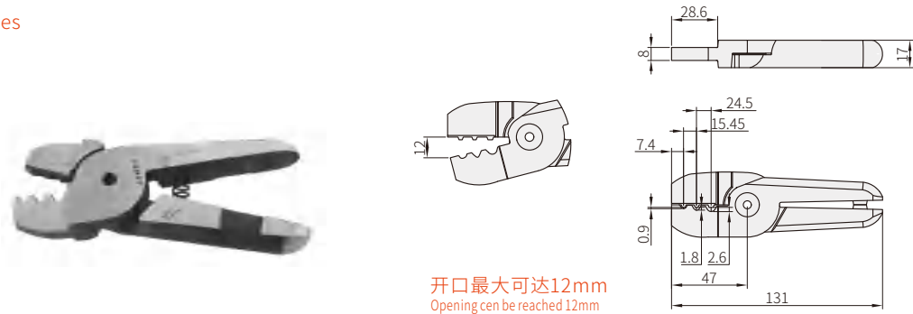
压线钳 Crimping pliers
