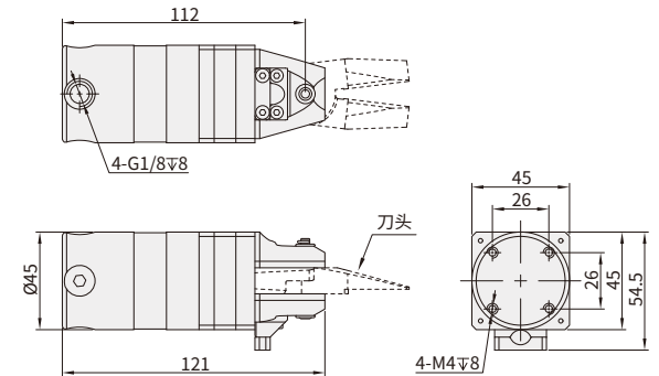
MD-20D气剪本体
