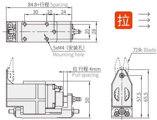
NL-10A气剪本体
