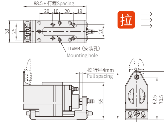
NL-15A气剪本体
