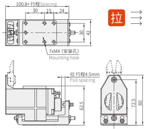
NL-25A气剪本体
