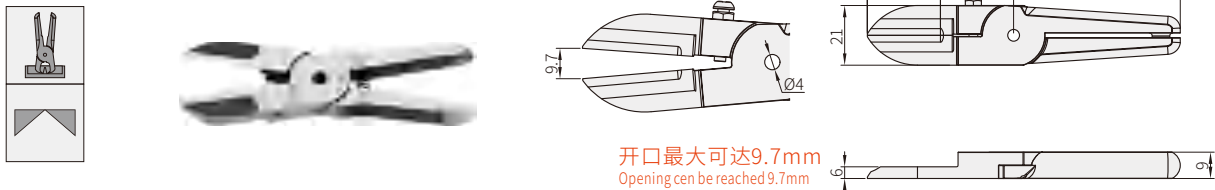
塑胶水口顶切平嘴钳(加长) Nipping blade(long)
