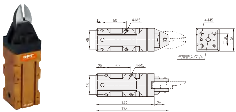
NF-230T气剪本体
