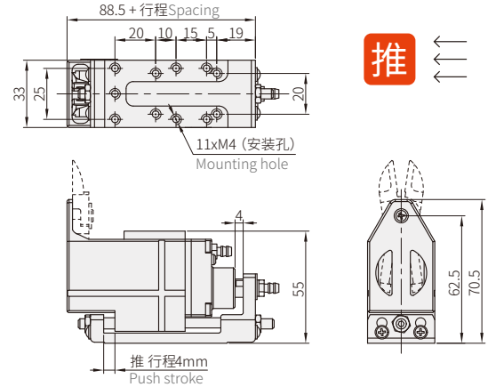
NL-15AR气剪本体
