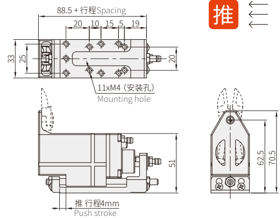
NL-15BR气剪本体
