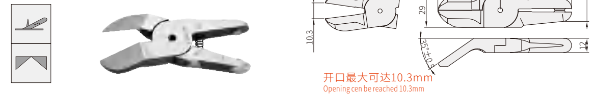
塑胶水口顶切斜嘴钳 Bevel Blade
