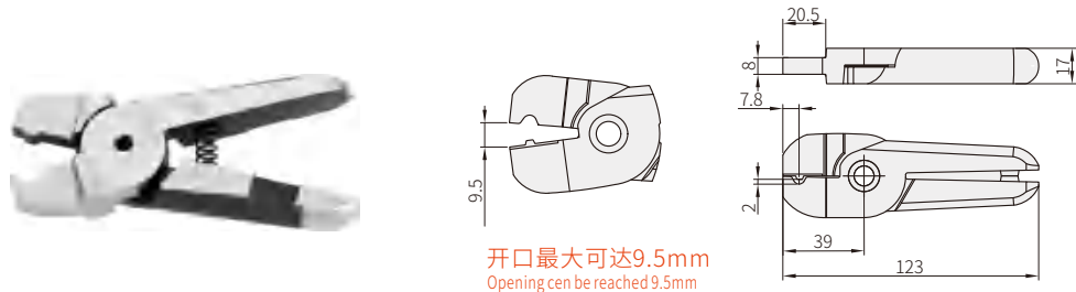
压线钳 Crimping pliers
