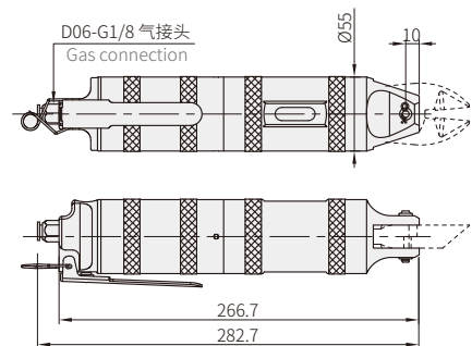
TS-35P气剪本体
