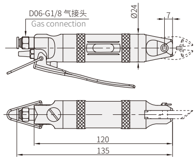
TS-3A气剪本体
