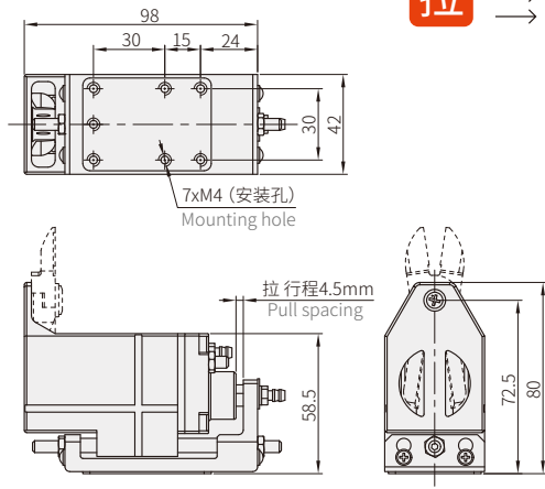
NL-25B气剪本体
