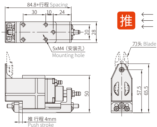
NL-10AR气剪本体
