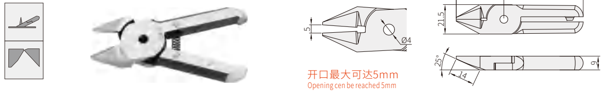
金属尖头斜嘴钳 Sharp bevel blade
