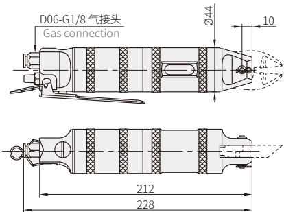
TS-25P气剪本体
