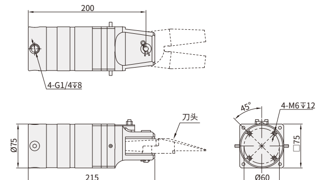
MD-50D气剪本体
