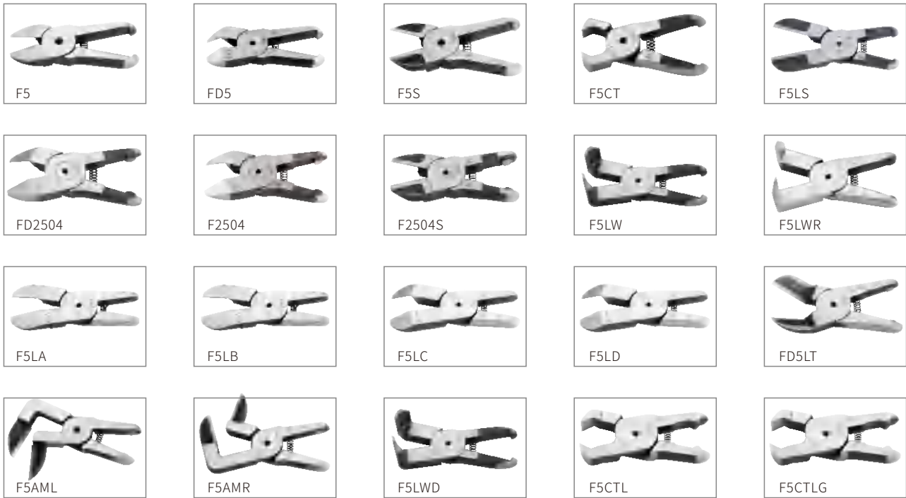
塑胶专用剪刀头 Adapter blade
