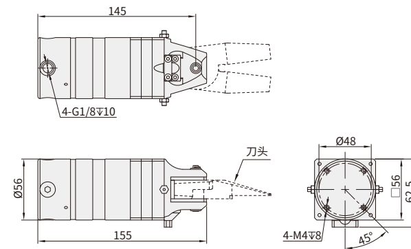
MD-30D气剪本体
