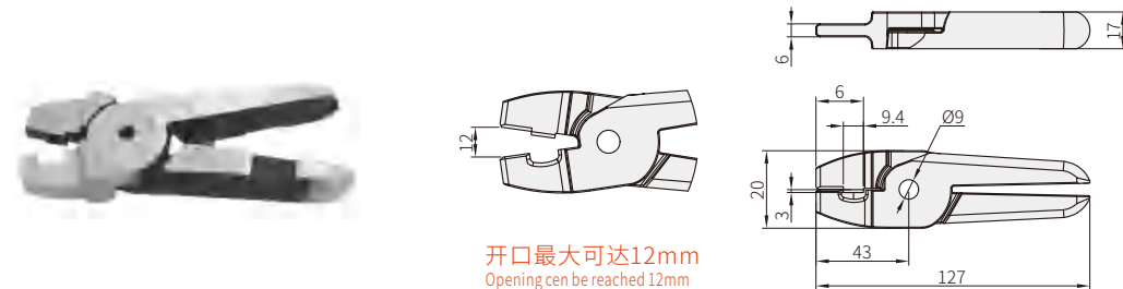
压线钳 Crimping pliers
