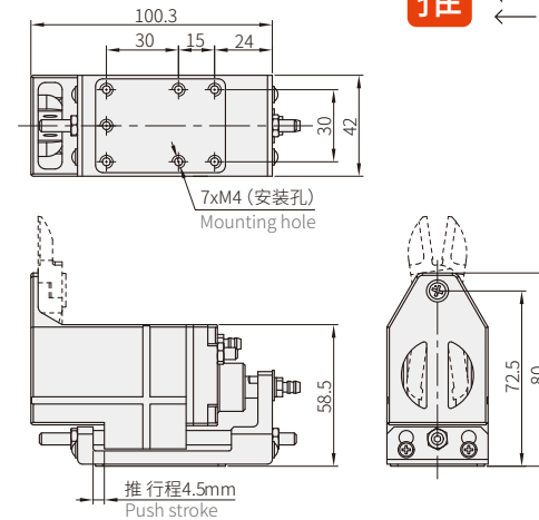
NL-25BR气剪本体
