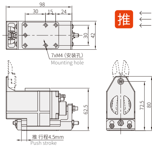
NL-25AR气剪本体
