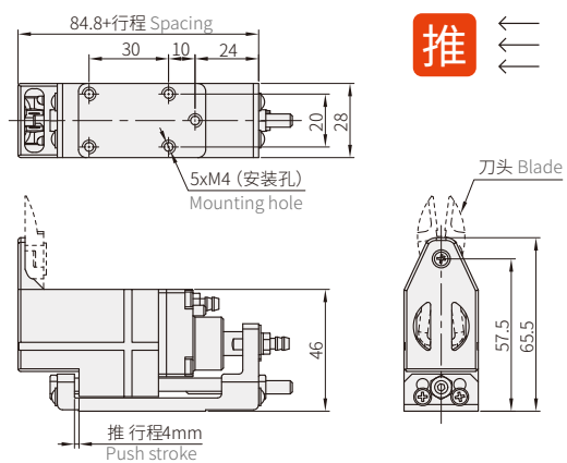
NL-10BR气剪本体
