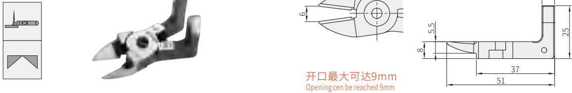
圆头平嘴钳 Round flat edge blade
