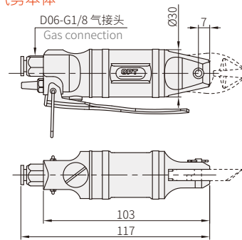
TS-5气剪本体
