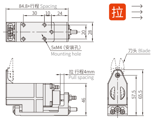
NL-10B气剪本体
