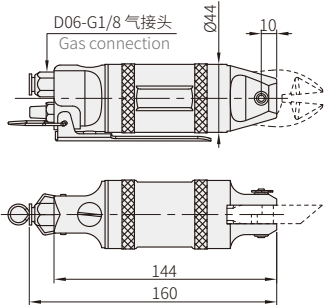
TS-20气剪本体
