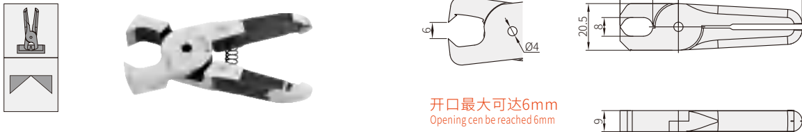
塑胶水口顶切平嘴钳 Nipping blade
