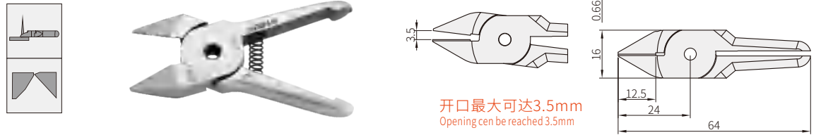
金属尖头斜嘴钳 Sharp bevel blade
