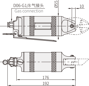
TS-30气剪本体
